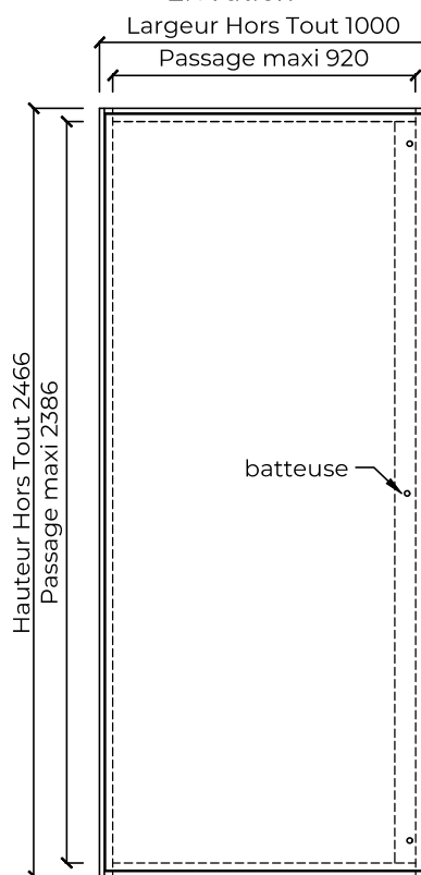
Élévation
